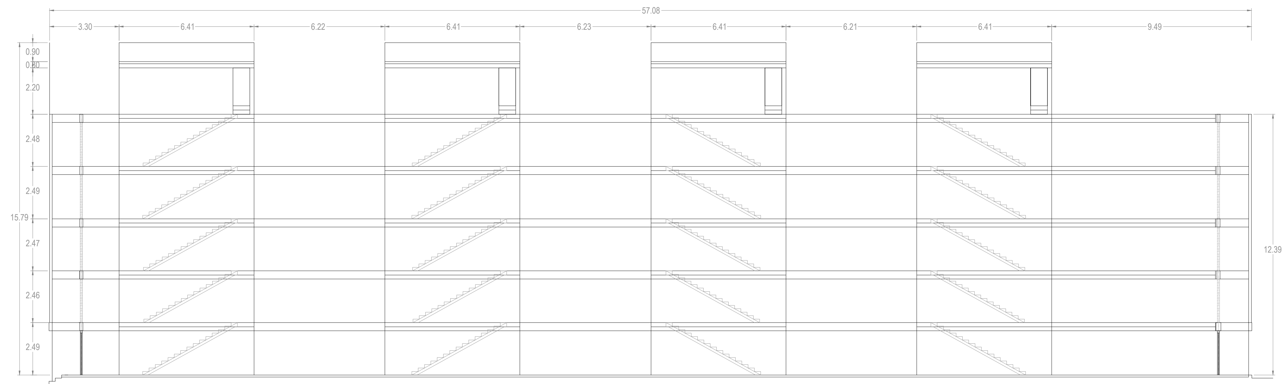
CORTE DE ELEVACION DE ESCALERAS Y AREAS COMUNES
